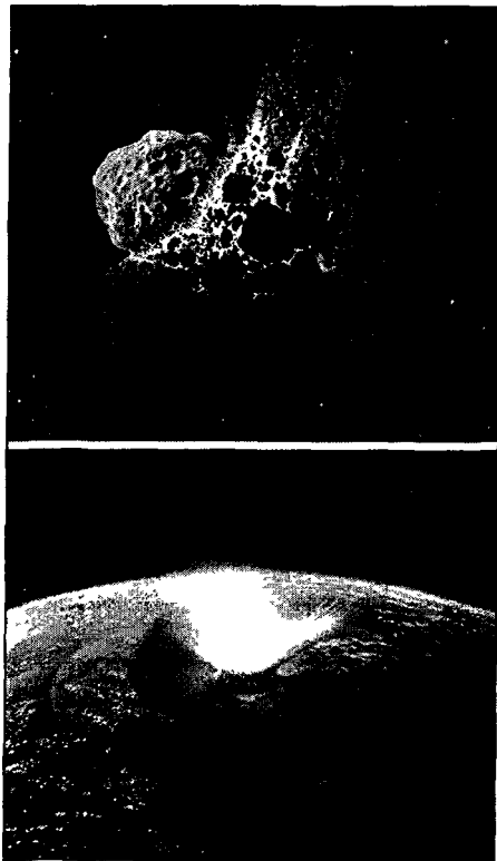
Рис. 21. Образовавшиеся в космосе астероиды при падении на нашу планету сильно изменяли климат Земли
