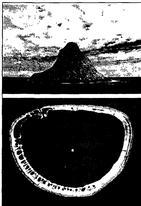
Рис. 41. Кальдера на острове в Восточном Средиземноморье
