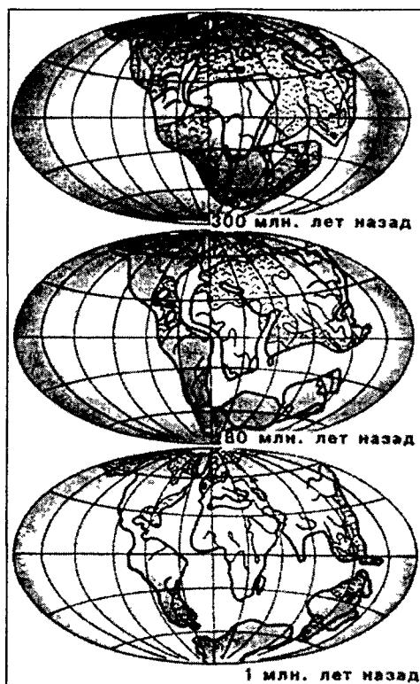
Рис. 34. Так, по утверждению некоторых ученых, происходили этапы раскола Пангеи
