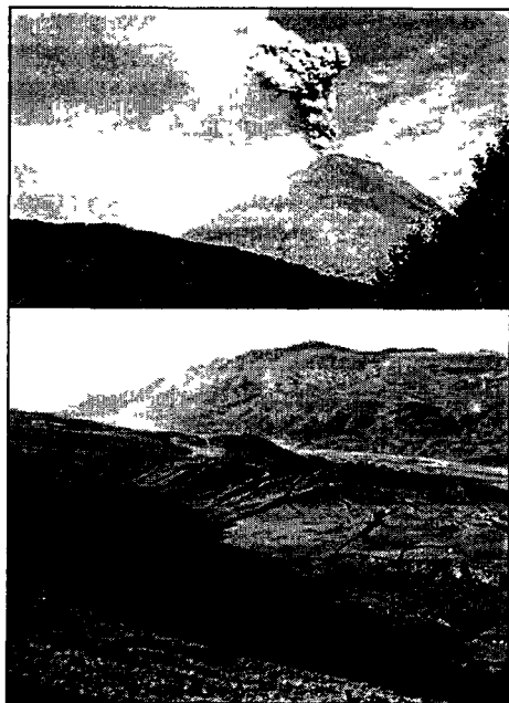
Рис. 78. Извержение вулкана — источник сильнейших явлений в литосфере, атмосфере и геокосмосе (вверху). Глубокие трещины в земной коре — последствия мощного землетрясения (внизу)
