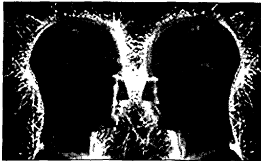
Рис. 58. Взаимодействие электрических полей
